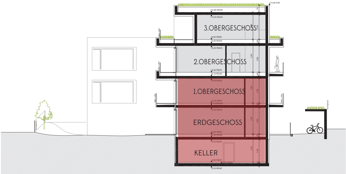
SYSTEMSCHNITT
